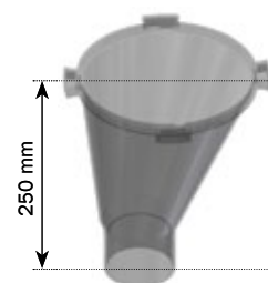
Bottom for VD5 Article nr. 0221-921
