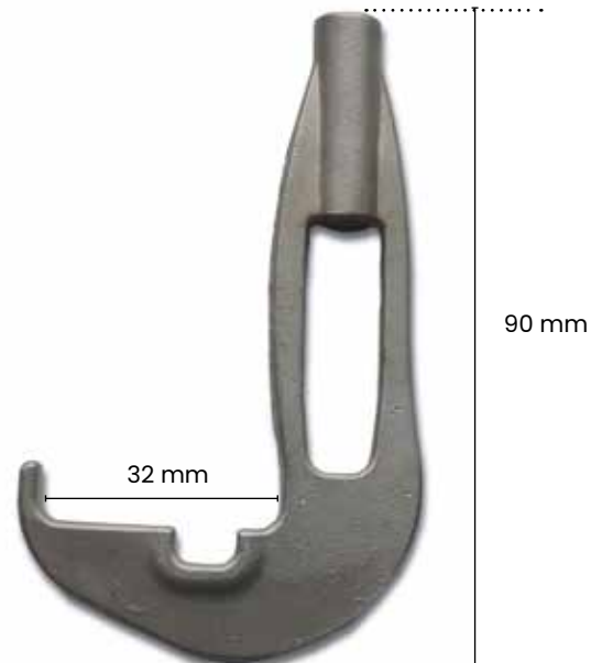
Anker til plastlameller Varenr. 30847
