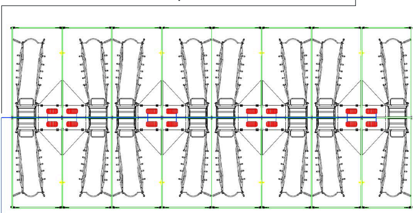
Installation af 16 Master Heater lamper med Multi kontakt A16.
