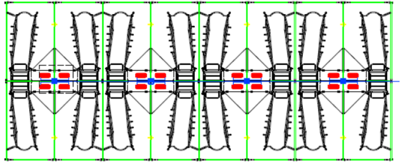
Installation af 16 Master Heater med 8 Dobbelt kontakter
