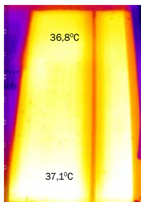
Termografisk varmefordeling for polymervarmeplade
