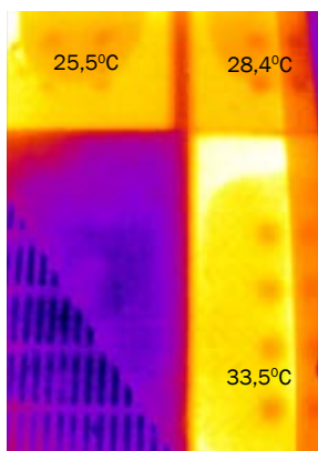
Termografisk varmefordeling for plastvarmeplade
