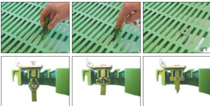
Montage Rautendübel - Artikelnr. 18958
